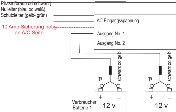
2 Batteriebanken Modell zum Laden von 2 separaten Batteriebanken als 2 x 12 v isoliert, oder kann zum Laden 1 Batterie zusammengeschlossen werden
